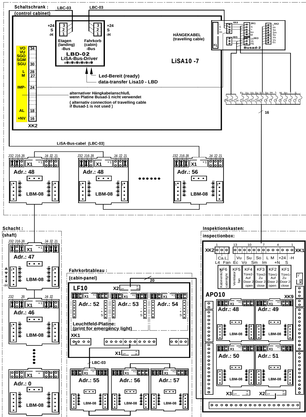
Blockschaltbild LiSA-Bus-System :
